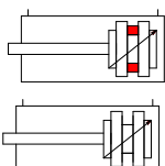
Doppio effetto magnetico ammortizzato Double acting magnetic cushioned
