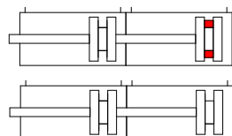
Tandem doppia spinta D.E.M. Double thrust tandem D.A.M.
