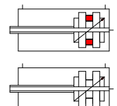
Doppio effetto magnetico ammortizzato con stelo cavo Double acting magnetic cushioned with hollow rod
